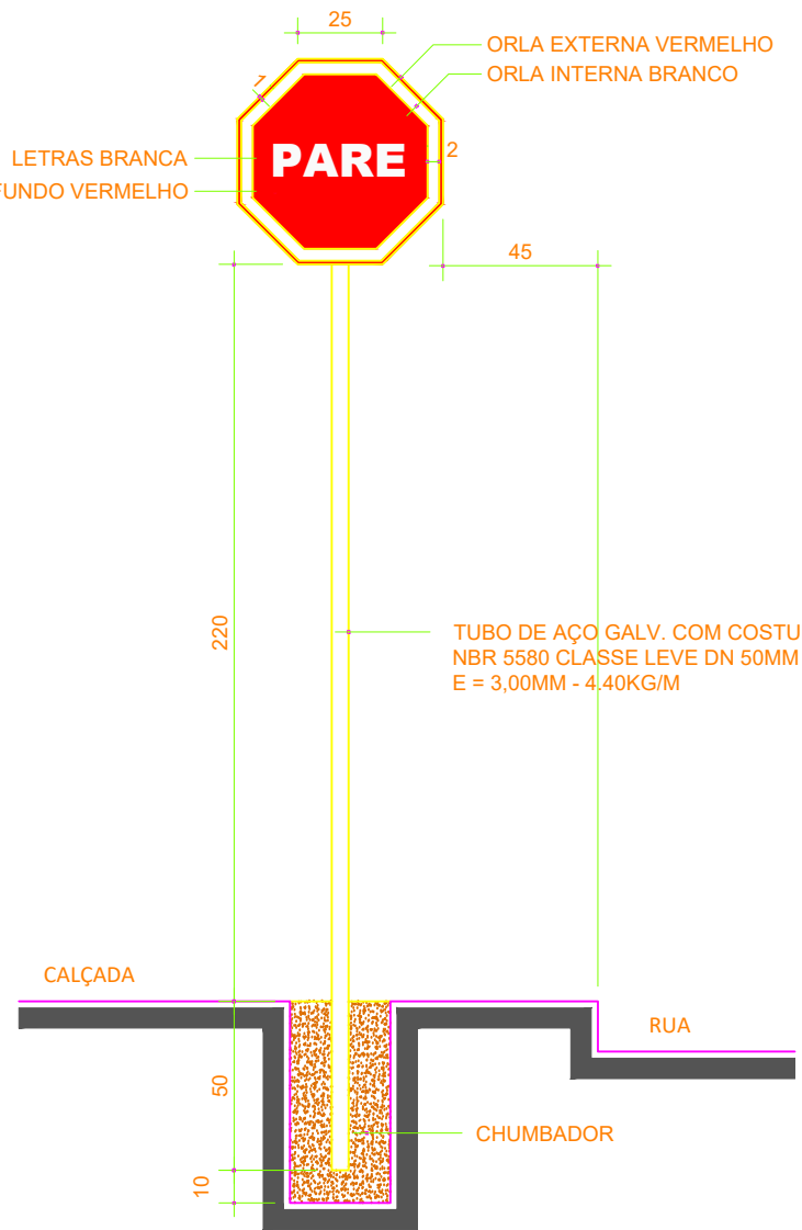
DETALHE PLACA PARE - R-1
