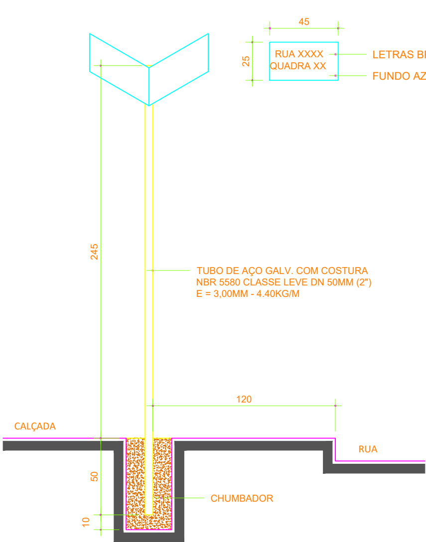
DETALHE PLACA DENOMINATIVAS DE LOGRADOURO PÚBLICOS
