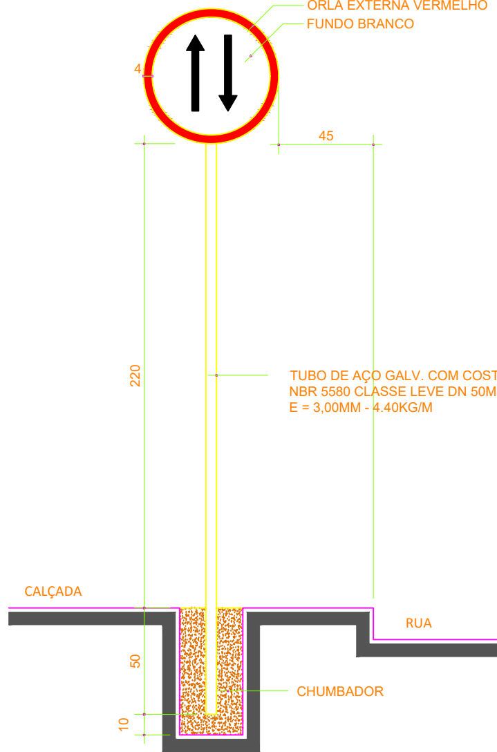
DETALHE PLACA R-28 SENTIDO DUPLO
