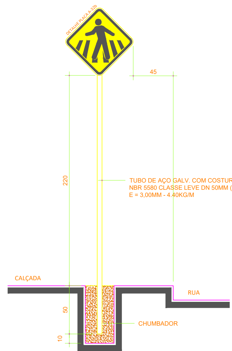
DETALHE PLACA A-32b
