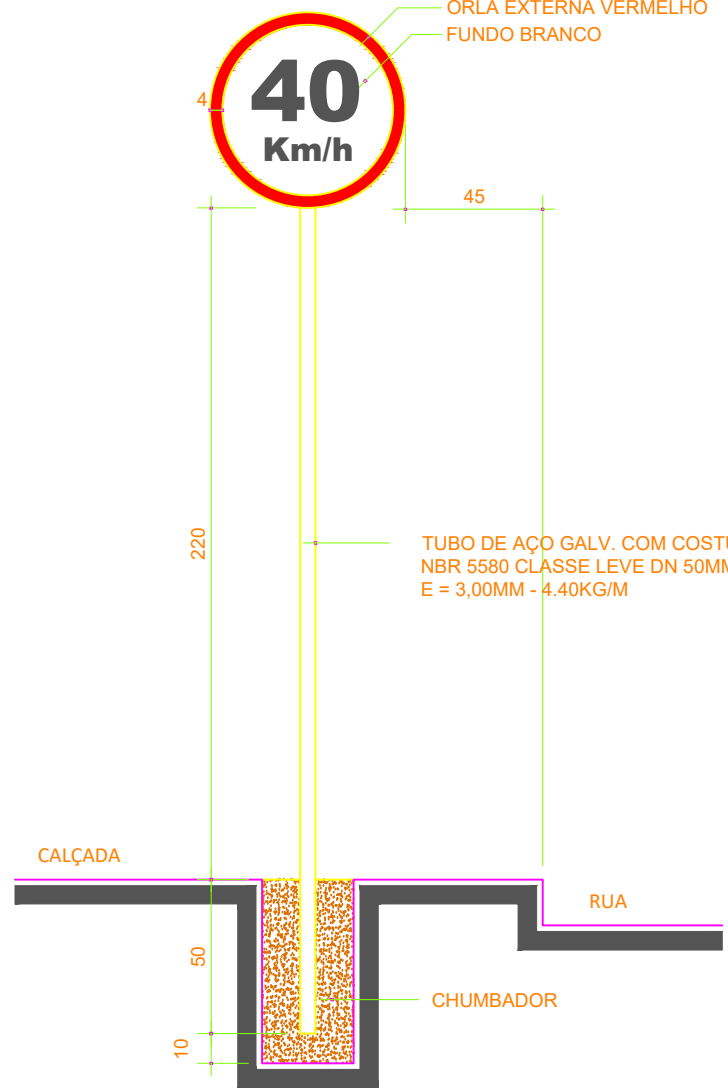
DETALHE PLACA VELOCIDADE MÁXIMA R-19 (40 Km/h)
